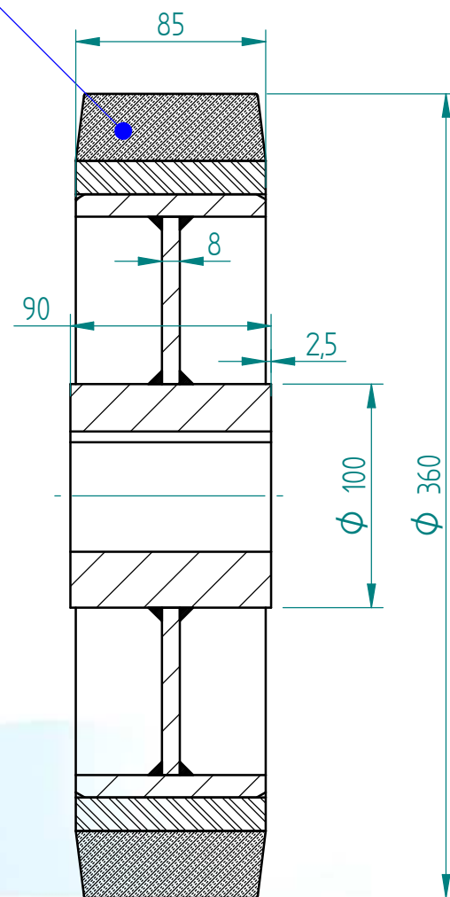
COUPE A-A 1:3
